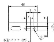
●取付金具下詳細図 (S=1/2) 左右共通
