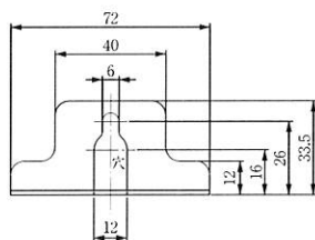
●取付金具上詳細図 (S=1/2)
