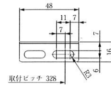
●取付金具下詳細図 (S=1/2) 左右共通
