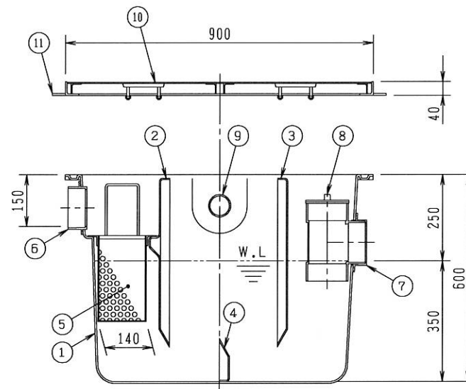
X-X断面図
