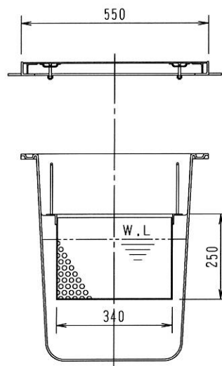
Y-Y断面図
