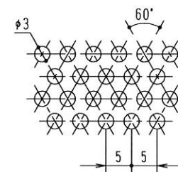
パンチングプレート打抜穴詳細
