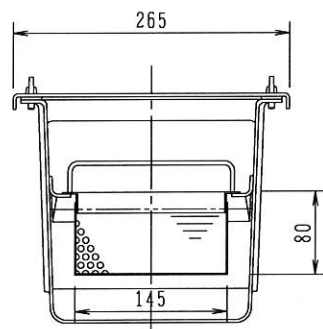
Y-Y断面図
