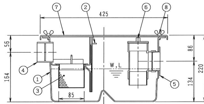
X-X断面図
